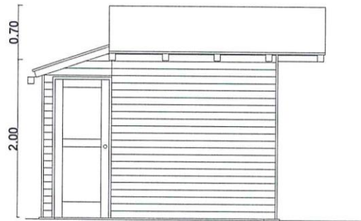
Varianta 2 (3x3) Pogled od strani
